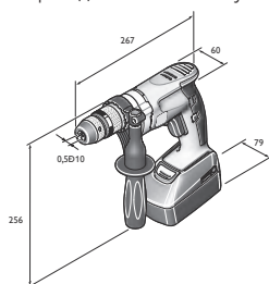
АВОП 6
