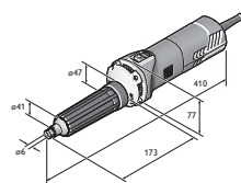
GSZ 8-90 PEL
