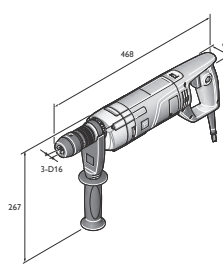
BOS 16-2
