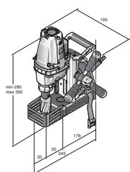
КВЕ 30
