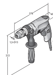
ВОП 10
