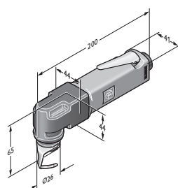
MOTlx 6-25
