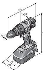
ASB 18 Q
