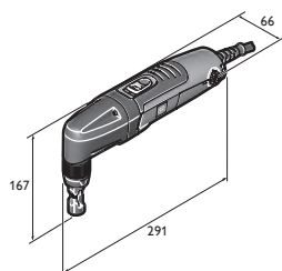
BLK 2.0 E
