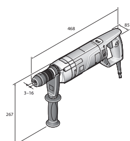
BOS 16
