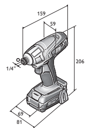
ASCD 12-100 W4C
