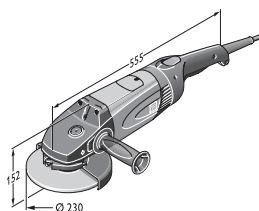
WSG 20-230 WSG 25-230
