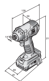
ASCD 12-150 W4C
