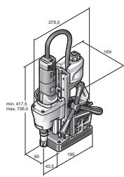
КВЕ 35
