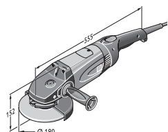
WSG 20-180 WSG 25-180
