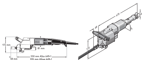
ASTx 649-1 ASTxe 649-1
