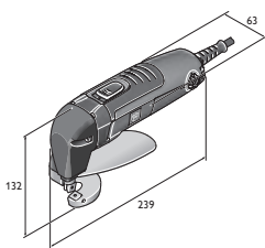
BLS 1.6 E
