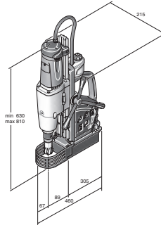
KBU 110-4 M
