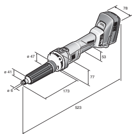
AGSZ 18-90 LBL
