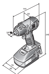
ASCD 18-300 W2
