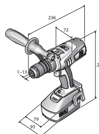
ASCM 18 QM
