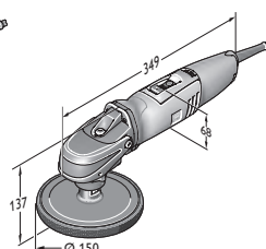
WPO 10-25 E
