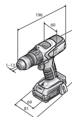
ASCM 12 Q
