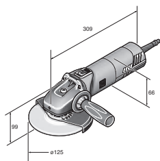
WSG 17-70 Inox
