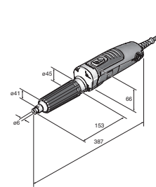
GSZ 4-90 EL
