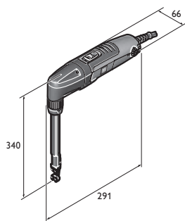
BLK 1.6 LE
