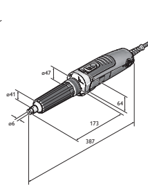
GSZ 4-280 EL
