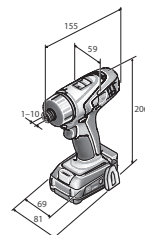
ABSU 12 W4
