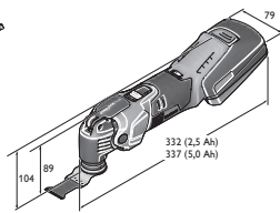
AMM 500
